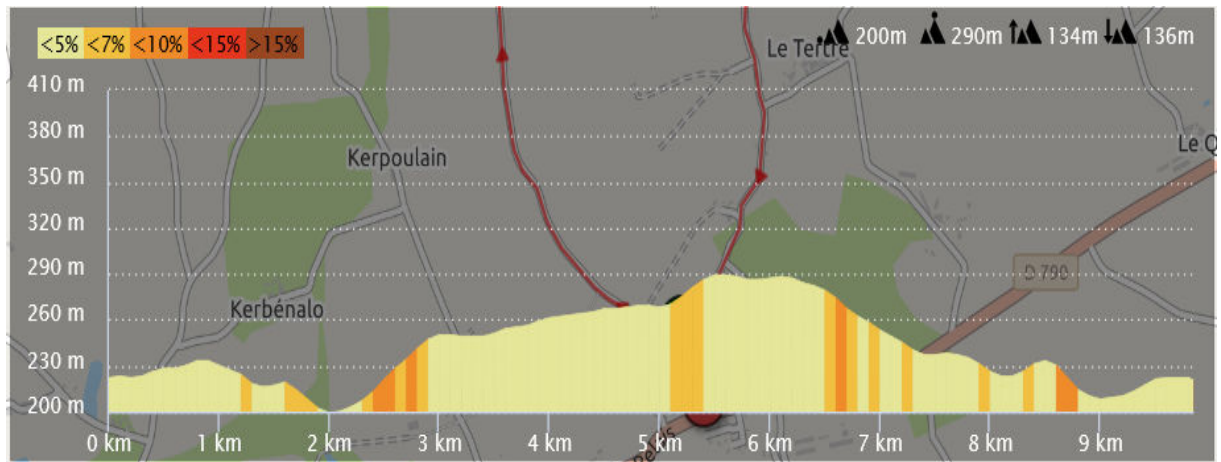
Profil du Circuit KBA Veranda line 2022
